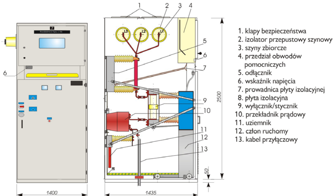
Elewacja i przekrój pola z wyłącznikiem
