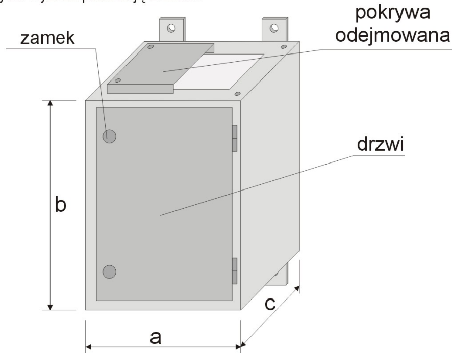
Widok skrzynki sterowniczej SST
