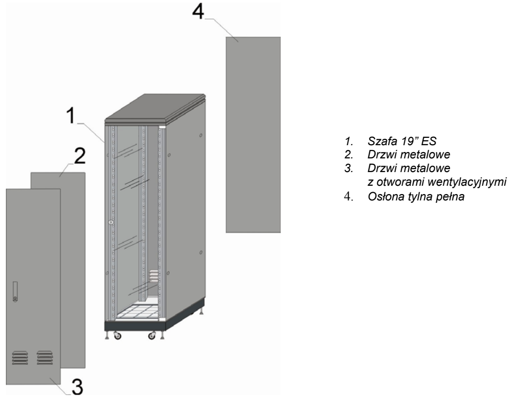
Szafa 19" ES z elementami wymiennymi
