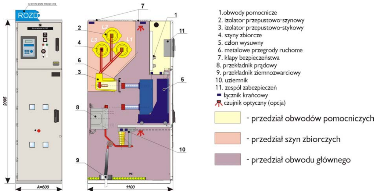
Przykład pola rozdzielnic D-12PT, D-17PT
